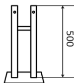
Закладная столба
