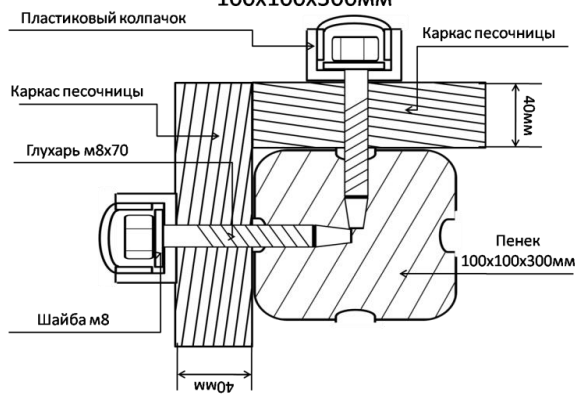
Крепления каркаса песочницы к пенку 100х100х300мм
