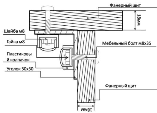
Крепления фанерных щитов с уголком 50х50
